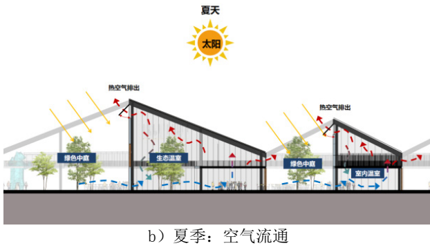
图9 节能示意图
